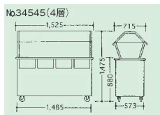
③ポータブルホットフードステーション (4槽) 94
