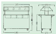
①ビュッフェ ホットフードステーション (4槽) 94
