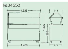
④ポータブルコールドフードステーション 94
