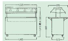
②ビュッフェ コールドフードステーション 94
