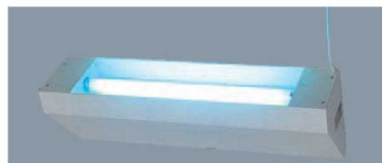
屋内用 ⑧シュアー粘着式捕虫器 ㍿ ページコード 商品コード 価格 MC-500 2-2058-0801 1128300 ¥35,000 外寸:575×132×H190 重量:2.0kg 電源:単相100V 50/60Hz 有効面積:30~45㎡ 誘虫ランプ:15W(FL-15BL) 電源コード:1.8m 電源スイッチ:「入」「切」スイッチ本体側面 粘着紙寸法:430×125 捕虫紙:1枚入り 捕虫紙MP-5001(10枚入) 2-2058-0802 1128310 ¥4,500 ㍿
