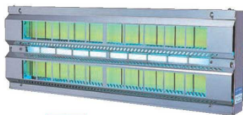
屋内用 ④ピオニー 捕虫器 ㍿ ページコード 商品コード 価格 F-200X型 2-2058-0401 4397000 ¥36,300 716×97×H236 重量:2.6kg(捕虫ランプ含む) 電源:単相100V 有効面積:40~60㎡ 誘虫ランプ:20W×1灯(FL-20SBL) 本体:18-8ステンレス製、インバーター方式 捕虫テープ2枚入 ※吊下げ、壁掛けタイプ ●害虫を落とすと必ずその場でキャッチし、捕虫テープの取り替えだけで、死がいの処理がワンタッチで衛生的です。 捕虫テープ(20枚入) 2-2058-0402 4265400 ¥6,000 ㍿
