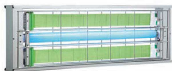
屋内用 ①捕虫器 ムシポン ㍿ ページコード 商品コード 価格 MPX-2000 2-2058-0101 5183300 ¥31,800 重量:2.4kg ●両面誘引型(両面とも捕虫紙に目隠しの無いもの) 捕虫紙 S-20(5枚入) 2-2058-0102 5183700 ¥1,500 ㍿
