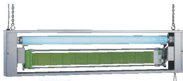
屋内用 ③捕虫器 ムシポン ㍿ ㍿ ㍿ ページコード 商品コード 価格 MP-301 2-2058-0301 8436200 ¥24,800 外寸:740×60×H175 重量:1.5kg 電源:単相100V 50Hz/60Hz 有効面積:50~80㎡ 誘虫ランプ:FL30SBL・1灯(30W) 材質:ステンレス 捕虫紙(5枚)1個人入り ●オールステンレスで錆びにくいも清潔 ●30Wインバーター使用で強力な誘引力 ●本体重量1.5kgと今までにない軽量化を実現 捕虫紙 S-20(5枚入) 2-2058-0302 5183700 ¥1,500 ㍿
