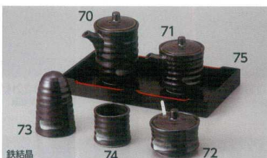
鉄結晶
