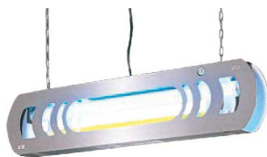
屋内用 ⑥シュアー捕虫器 ムシキャッチボン ㊦ ページコード 商品コード 価格 MC-400 3-2076-0601 1129300 ¥14,000 外寸:684×61×H157 ●紙でできた使い切り捕虫器(ケース・トレイのみ) ●煩わしい清掃が不要で捨てるゴミとして捨てられます。 ●屋内に侵入した虫を粘着液で一網打尽にします。 ●高電圧がなく安全。又、修理がいりません。 捕虫ケースセットMP-4001 3-2076-0602 1129310 ¥3,150 ㊦ (ケース4個、マジックテープ6個) 捕虫トレイセットMP-4002 3-2076-0603 1129320 ¥2,520 ㊦ (トレイ4個)
