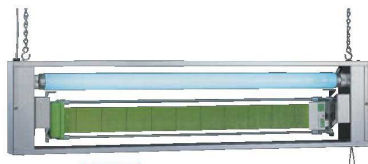
屋内用 ③捕虫器 ムシボン ㊦ ㊦A ページコード 商品コード 価格 MP-301 3-2076-0301 8436200 ¥24,800 外寸:740×60×H175 重量:1.5kg 電源:単相100V 50Hz/60Hz 有効面積:50~80㎡ 誘虫ランプ:FL30SBL・1灯(30W) 材質:ステンレス 捕虫紙(5枚)1個人入り ●オールステンレスで錆びにくい清潔 ●30Wインバーター使用で強力な誘引力 ●本体重量1.5kgと今までにない軽量化を実現 捕虫紙 S-20(5枚入) 3-2076-0302 5183700 ¥1,500 ㊦
