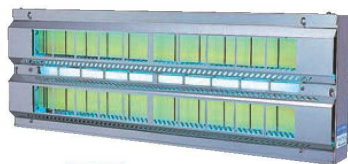
屋内用 ④ピオニー 捕虫器 ㊦ ページコード 商品コード 価格 F-200X型 3-2076-0401 4397000 ¥36,300 716×97×H236 重量:2.6kg(捕虫ランプ含む) 電源:単相100V 有効面積:40~60㎡ 誘虫ランプ:20W×1灯(FL-20SBL) 本体:18-8ステンレス製、インバーター方式 捕虫テープ2枚入 ※吊下げ、壁掛けタイプ ●害虫を落とさずその場でキャッチし、捕虫テープの取 り替えだけで、死がいの処理がワンタッチで衛生的です。 捕虫テープ(20枚入) 3-2076-0402 4265400 ¥6,400 ㊦
