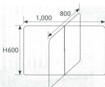
7-1222-1 (11024670) ¥9,800 クロスパーティション(3mm厚) AC 1,000×800×H600
