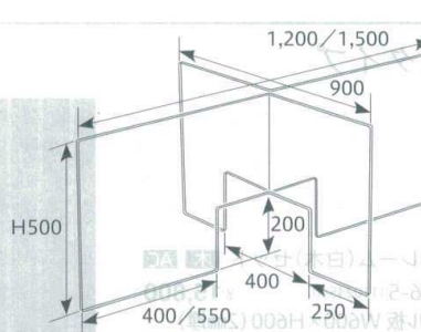
窓アリタイプ2枚と十字ストッパー使用例
