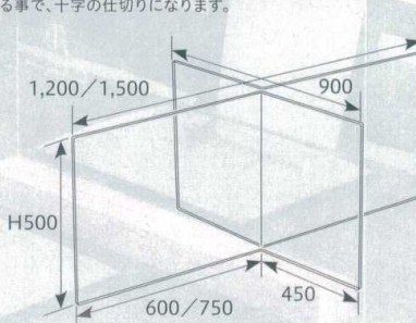
窓ナシタイプ2枚と十字ストッパー使用例
