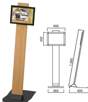
② そうきゅう PA-A4Y
