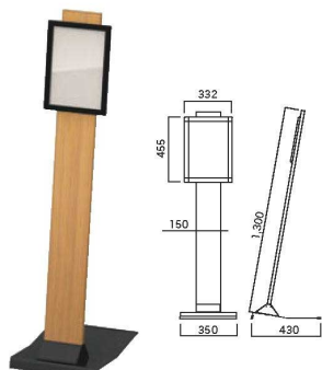
① そうきゅう PA-A4T
